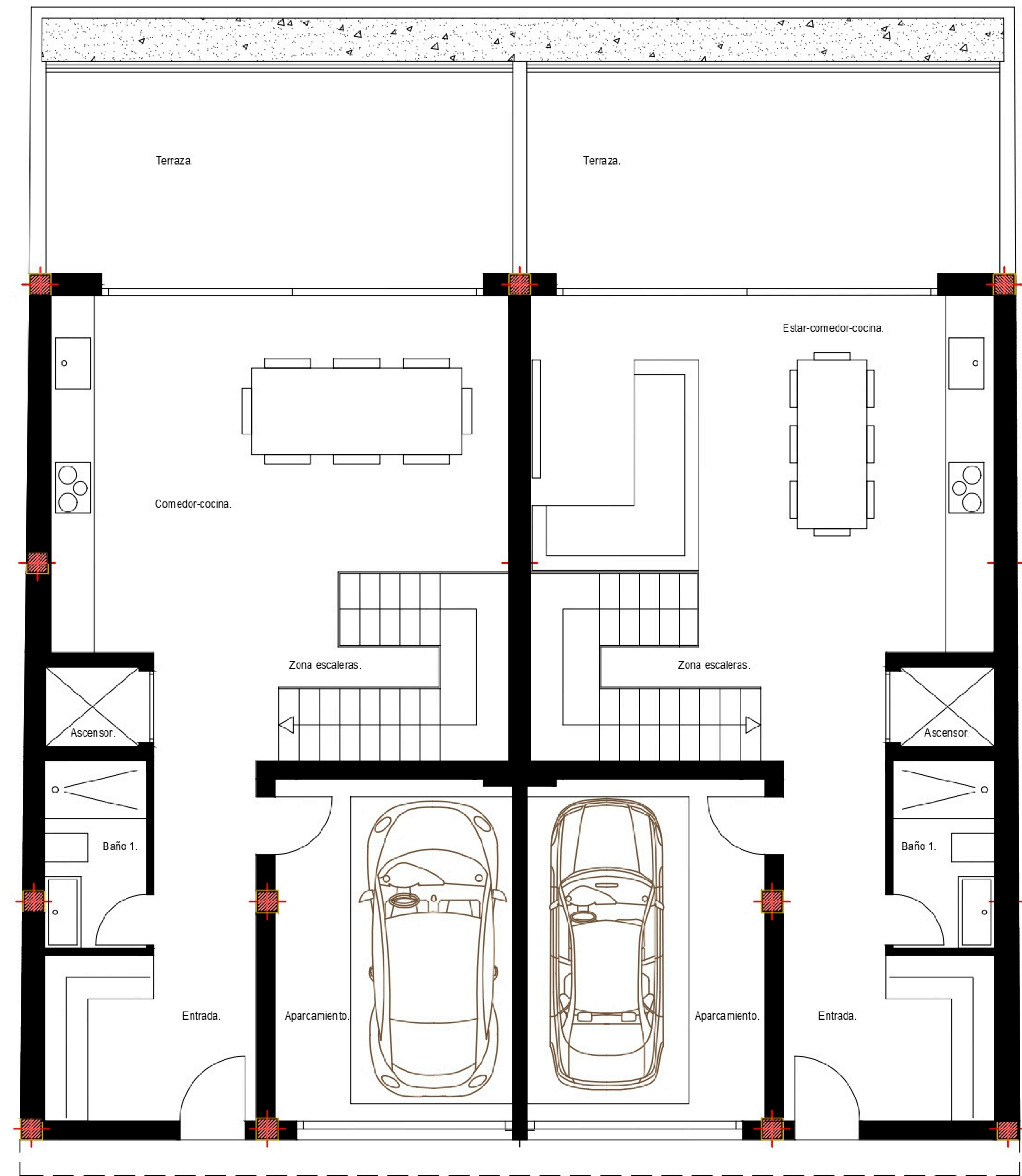
PLANTA BAJA.
