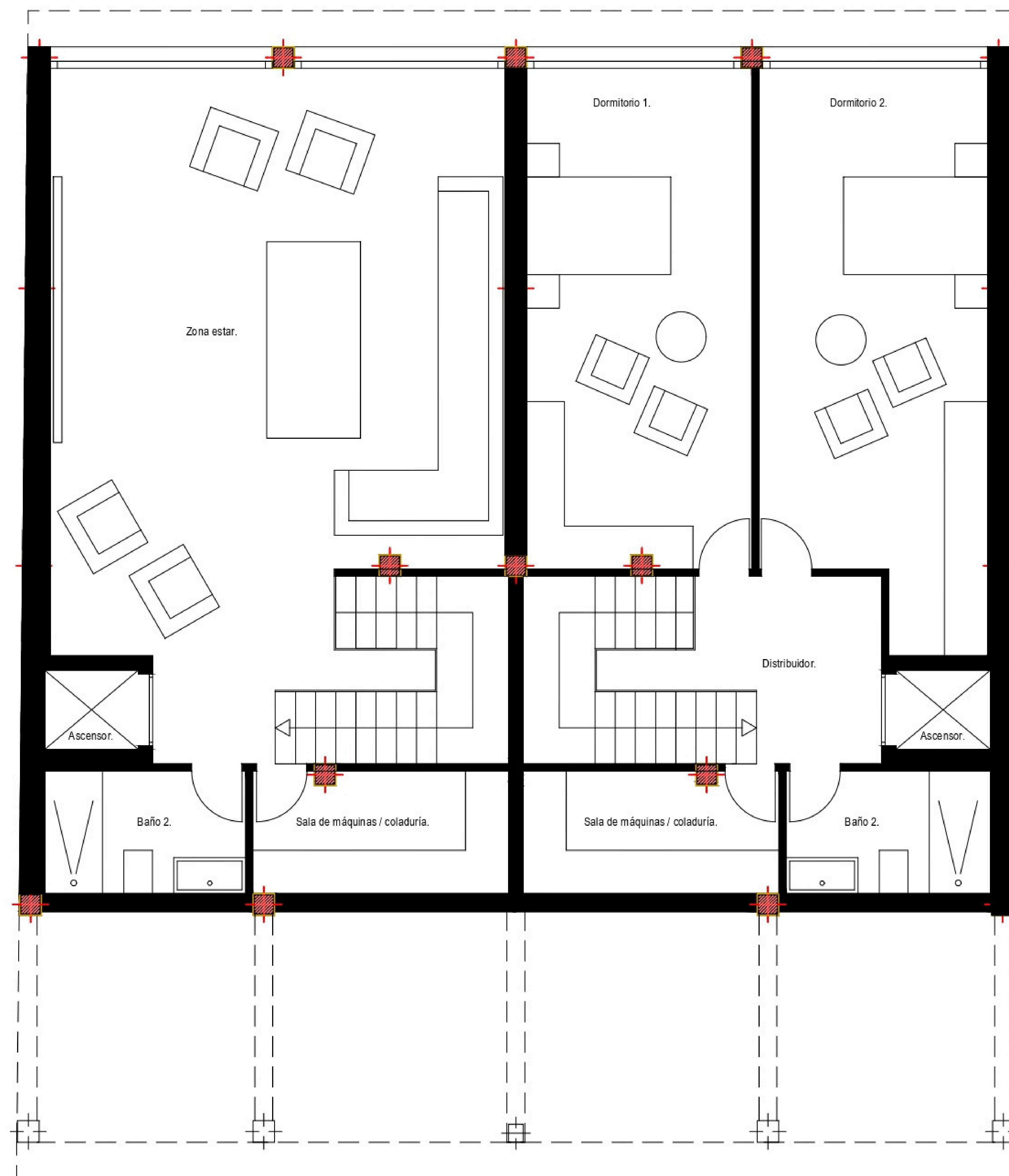
PLANTA -1.
